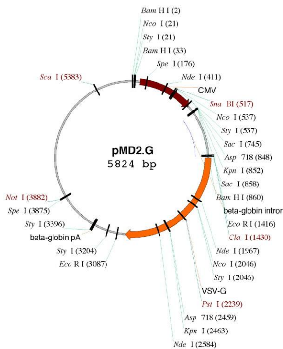
شکل ۲: وکتور pMD2G (۱۴)
