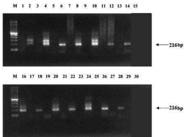
شکل ۱: ژل حاصل از آزمون RT-PCR در نمونه‌های مورد بررسی. نمونه شماره ۱۶ کنترل مثبت و نمونه شماره ۱۷ کنترل منفی می‌باشد. مارکر مورد استفاده، مارکر ۱۰۰ bp، ساخت شرکت فرمتاز است. مشاهده باند ۲۱۶ bp نشان‌دهنده مثبت بودن نمونه‌های مورد بررسی می‌باشد.
