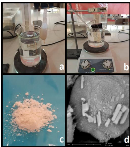
شکل ۱: (a و b) مراحل لابر اتواری تهیه پودر میکروبیزه ابریشم طبیعی از پیله کرم ابریشم. c: پودر ابریشم طبیعی میکروبیزه. d: تصویر میکروسکوپ الکترونی از پودر ابریشم طبیعی با میکروسکوپ SEM (PHENOM PROX)
