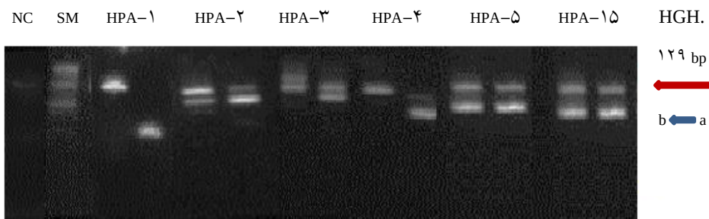
شکل ۱: باندهای حاصل از الکتروفورز محصولات PCR مربوط به ژن‌های مختلف HPAs در یکی از بیماران. در این شکل طول باند HPA-1:90 bp/ HPA-2:258 bp/ HPA-3: 367 bp/ HPA-4:126 bp/ HPA-5:250 bp/ HPA-15:225 bp است و NC در چاهک اول کنترل منفی می‌باشد.
