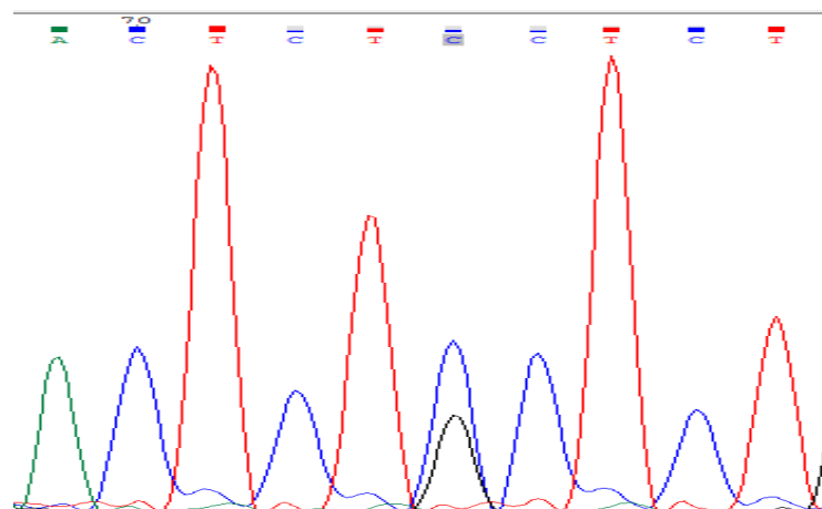
شکل ۵: کروماتوگراف حاصل از تعیین توالی اگزون ۵ ژن RHCE با استفاده از نرم افزار Chromas. در این نمونه در نوکلئوتید ۶۷۶، باز C و G وجود دارد که سبب می‌شود ژنوتیپ این نمونه به صورت هتروزیگوت RHCE*E/e باشد.
