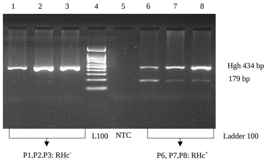
شکل ۲: الکتروفورز محصولات PCR-SSP مربوط به اگزون ۲ آلل RhC بر روی ژل آگارز ۲٪. نمونه بیماران در ستون‌های ۱، ۲ و ۳ منفی (تنها باند هورمون رشد دیده می‌شود) و نمونه بیماران در ستون‌های ۴، ۵ و ۶ مثبت (علاوه بر باند مربوط به هورمون رشد باند اختصاصی RhC به طول ۱۷۹ bp مشاهده می‌شود) می‌باشند، ردیف ۵: کنترل منفی آغازگر
