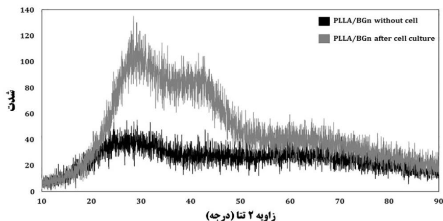
شکل ۲: الگوی پراش پرتو ایکس نانودار بست. نتیجه حاصل از بررسی پرتو ایکس نانو دار بست کامپوزیتی پلی‌ال‌لاکتیک اسید حاوی نانو ذرات شیشه زیست فعال (PLLA/BGn) ۴۵S۵ قبل از کشت سلول و پس از ۱۴ روز تمایز استخوانی سلول‌های بنیادی مزانشیمی
