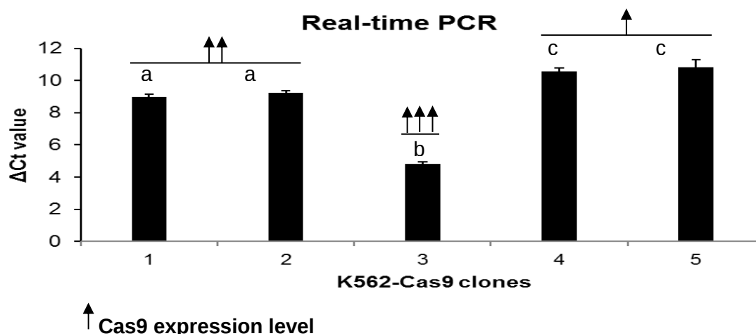
شکل ۷: نمایش منحنی‌های تکثیر و ذوب در واکنش Real-time PCR. (الف) منحنی‌های تکثیر رونوشت ژنهای B2M و کلون‌های بیان‌کننده Cas9 ، (ب) منحنی‌های ذوب رونوشت ژنهای B2M و Cas9 . (ج) مقایسه بیان ژن Cas9 در ۵ کلون مختلف جدا شده سلول K562-Cas9. کلون‌های آنالیز شده از لحاظ میزان بیان Cas9 به سه گروه با بیان کم (۴ و ۵)، متوسط (۱ و ۲) و بالا (۳) تقسیم شدند. a، b و c معنادار بودن آماری داده‌ها را نشان می‌دهند ( p < 0.0001 ).
