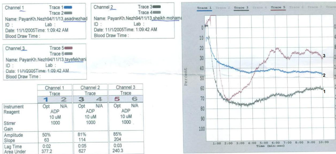
نمودار ۲: نمودار اگرگاسیون پلاکت‌ها در مواجهه با آگونیست ADP، منحنی‌های شماره ۲ و ۳ تجمع پلاکتی گروه بیماران قلبی واجد پلاک آنرواسکلروتیک بدون مصرف داروی آنتاگونیست و منحنی شماره یک کنترل می‌باشد.
