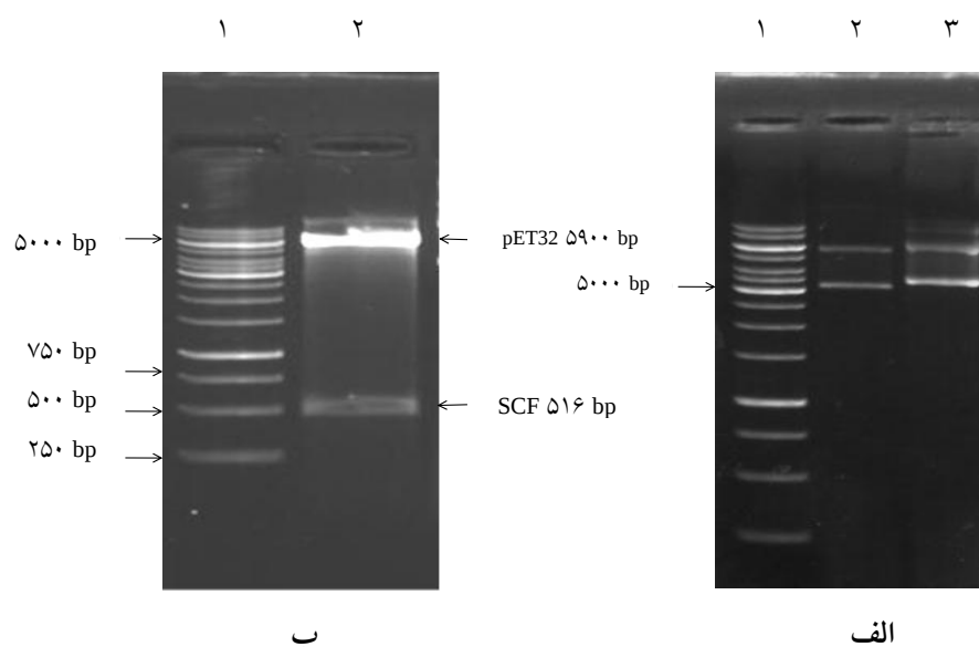
شکل ۳: الف) الکتروفورز پلاسمید نوترکیب در مقایسه با پلاسمید pET-32 کنترل؛ الکتروفورز پلاسمید استخراج شده از کلونی مثبت (ستون ۳) در کنار پلاسمید pET-32 به عنوان کنترل (ستون ۲) با نشان دادن تأخیر در حرکت بر روی ژل آگارز ۱/۵٪، نوترکیب ارزیابی شد. ستون ۱ شاخص اندازه مولکولی ۱ کیلوبازی است. ب) الکتروفورز محصول واکنش هضم آنزیمی وکتور نوترکیب؛ ستون ۱ شاخص اندازه مولکولی ۱ کیلوبازی، ستون ۲ جدا شدن توالی رمزکننده SCF به طول ۵۱۶ جفت باز از وکتور نوترکیب که با پیکان مشخص شده است را نشان می‌دهد.
