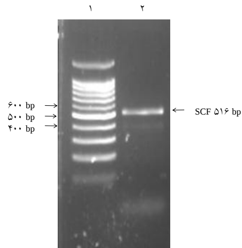
شکل ۲: الکتروفورز محصول PCR توالی رمزکننده فاکتور سلول بنیادی بر روی ژل آگارز ۲٪ در بافر TAE؛ در ستون اول شاخص اندازه مولکولی ۱۰۰ جفت بازی و در ستون دوم باند ۵۱۶ جفت بازی محصول تکثیر توالی رمزکننده SCF به وسیله آنزیم pfu DNA polymerase و در حضور آغازگرهای اختصاصی با پیکان نشان داده شده است.
