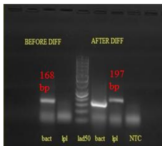
شکل ۳: نمای ژل الکتروفورز بعد از الکتروفورز محصول PCR: (۱) beta actin قبل از تمایز، (۲) LPL قبل از تمایز (۳) سایز مارکر (۴) ۵۰ bp beta actin بعد از تمایز (۵) LPL بعد از تمایز (۶) NTC
