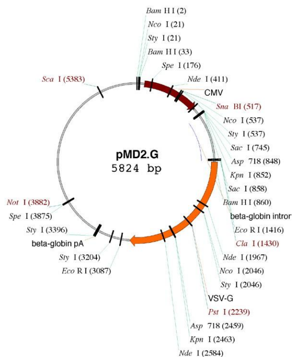
شکل ۲: وکتور pMD2.G (۱۴)
