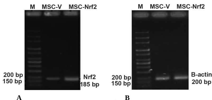
شکل ۲- A: بررسی بیان ژن Nrf2 در دو گروه سلولی تحت مطالعه با روش RT-PCR. M: مارکر (100 bp) DNA، ردیف MSC-V ، MSCs : ترانسفکت شده با پلاسמיד خالی، ردیف MSC-Nrf2 ، MSCs ترانسفکت شده با پلاسמיד pcDNA3.1-Nrf2 . گروه MSC-Nrf2 این ژن را بیشتر بیان کرد ( p < 0.01 ). B: بررسی بیان ژن بتا کتین ( \beta -actin) در دو گروه سلولی تحت مطالعه. بیان بتا کتین در دو گروه اختلاف معنادار نداشت.
