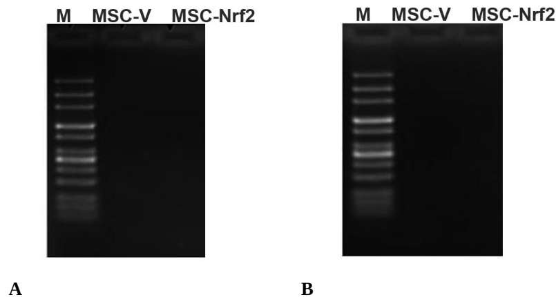
شکل ۴- A: بررسی بیان ژن HO-1 در دو گروه سلولی تحت مطالعه با روش RT-PCR. M: مارکر (۱۰۰ bp) DNA، ردیف MSC-V: MSCs: ترانسفکت شده با پلاسمید خالی، ردیف MSC-Nrf2: MSCs: ترانسفکت شده با پلاسمید pcDNA3.1-Nrf2 . هر دو گروه این ژن را بیان نکردند. B: بررسی بیان ژن NQO1 در دو گروه سلولی تحت مطالعه با روش RT-PCR. M: مارکر (۱۰۰ bp) DNA، ردیف MSC-V: MSCs: ترانسفکت شده با پلاسمید خالی، ردیف MSC-Nrf2: MSCs: ترانسفکت شده با پلاسمید pcDNA3.1-Nrf2 . هر دو گروه این ژن را بیان نکردند.
