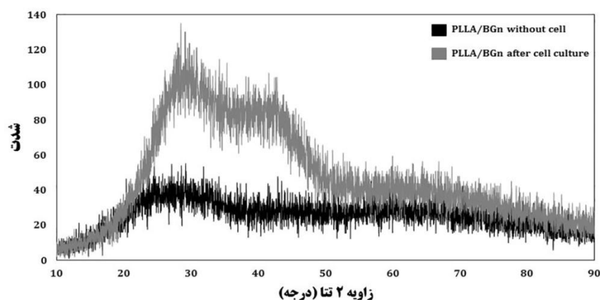
شکل ۲: الگوی پراش پرتو ایکس نانودار بست. نتیجه حاصل از بررسی پرتو ایکس نانو دار بست کامپوزیتی پلی‌الاکتیک اسید حاوی نانو ذرات شیشه زیست فعال (PLLA/BGn) ۴۵۵۵ قبل از کشت سلول و پس از ۱۴ روز تمایز استخوانی سلول‌های بنیادی مزانشیمی
