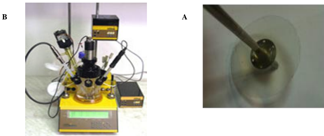
شکل ۱: A: هم‌زن fish tail به کار رفته در بیوراکتور. B: بیوراکتور سوسپانسیونی
