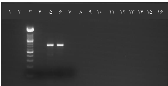
شکل ۱: الکتروفورز محصولات PCR semi-nested مربوط به پاروویروس B19 بر روی ژل آگارز ۲ درصد. ستون‌های ۱ و ۲ کنترل منفی، ستون ۳ ladder (نشانگر ۱۰۰ bp با علامت تجاری Roche®)، ستون‌های ۵ و ۶ کنترل مثبت (با طول باند ۷۱۷bp)، ستون ۴ و ۷ به بعد نشانگر PCR نمونه سرم اهداکنندگان خون می‌باشد.
