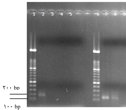
شکل ۶: نتیجه RT-PCR ژن Cas9 چاهک ۱: نشانگر وزن مولکولی ۱۰۰ جفت بازی، چاهک ۲: تکثیر رونوشت Cas9 از نمونه سلول K562 ترانسفکت شده، چاهک ۳: نمونه سلول K562 ترانسفکت نشده، چاهک ۴: محصول PCR بدون اضافه کردن cDNA (کنترل منفی)، چاهک ۵: نمونه RTminus (بررسی عدم وجود آلودگی DNA) از سلول ترانسفکت شده. چاهک ۶: نشانگر وزن مولکولی ۱۰۰ جفت بازی، چاهک ۷: تکثیر قطعه B2m از نمونه سلول K562 ترانسفکت شده. چاهک ۸: تکثیر قطعه B2m از نمونه سلول K562 ترانسفکت نشده، چاهک ۹: محصول PCR بدون cDNA الگو (کنترل منفی)
